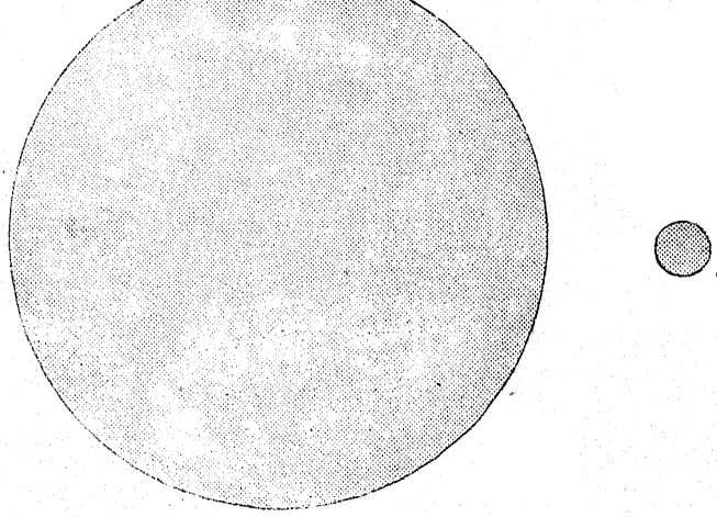
चित्र ४६—बृहस्पति और पृथ्वी की तुलना। पृथ्वी कितनी छोटी है! [सौर-परिवार से
